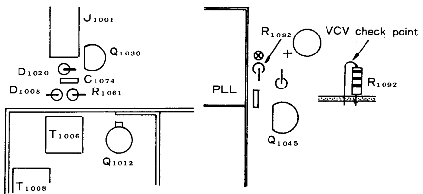
PLL 回路調整箇所
