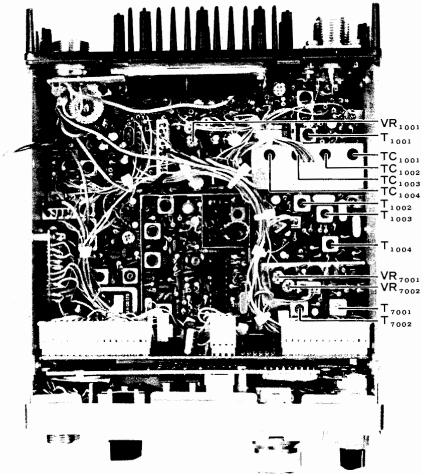
受信部調整個所
